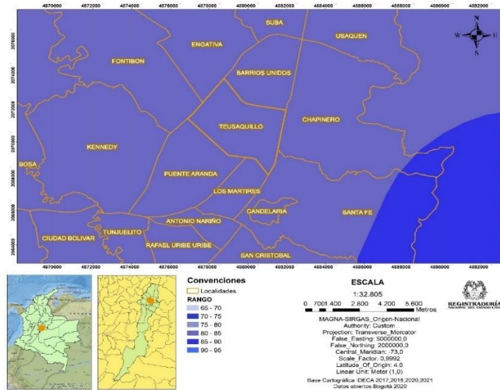
Figura 10. Temperatura media mensual
