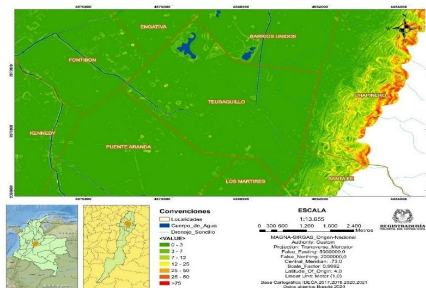
Figura 6. Pendientes Localidad de Teusaquillo
